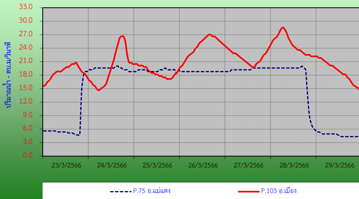
กราฟแสดงปริมาณน้ำปิงรายชั่วโมงรอบวันที่ 12/2566 ที่สถานีแม่ น้ำปิง ( P.75) บ้านซ้อแล อ.แม่แตง และที่สถานีแม่ น้ำปิง (P.103) บ้านป่าซ่อยใต้ อ.เมือง จ.เชียงใหม่
